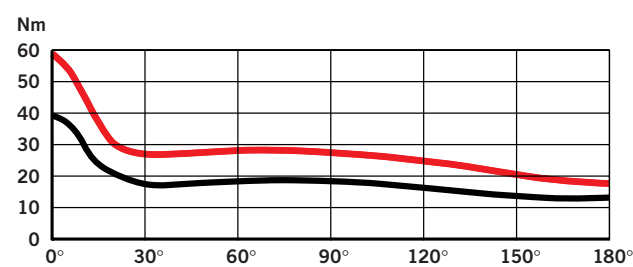
Diagrama de momentos DORMA TS 93 (Ajuste de la fuerza de cierre EN 5)
